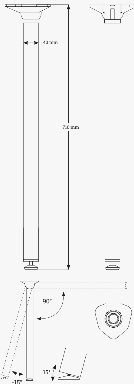
Technische Zeichnung
