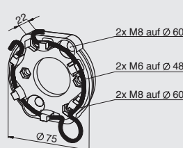
Markisen- und Universallager mit Gewinde
