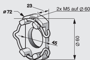
Kompakt- Antriebslager
