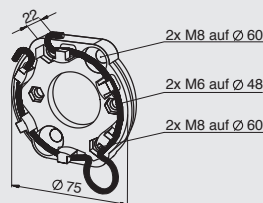
Markisen- und Universallager ohne Gewinde
