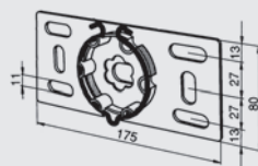
Flansch- Antriebslager
