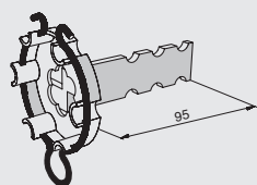
Eingipslager mit Federring
