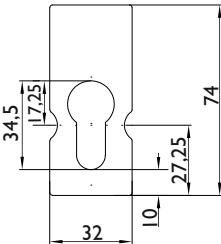
Bohrschutzplatte (selbstklebend)
