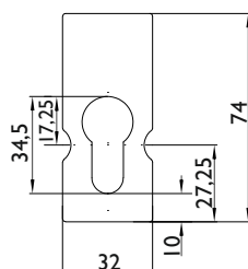
Bohrschutzplatte (selbstklebend)
